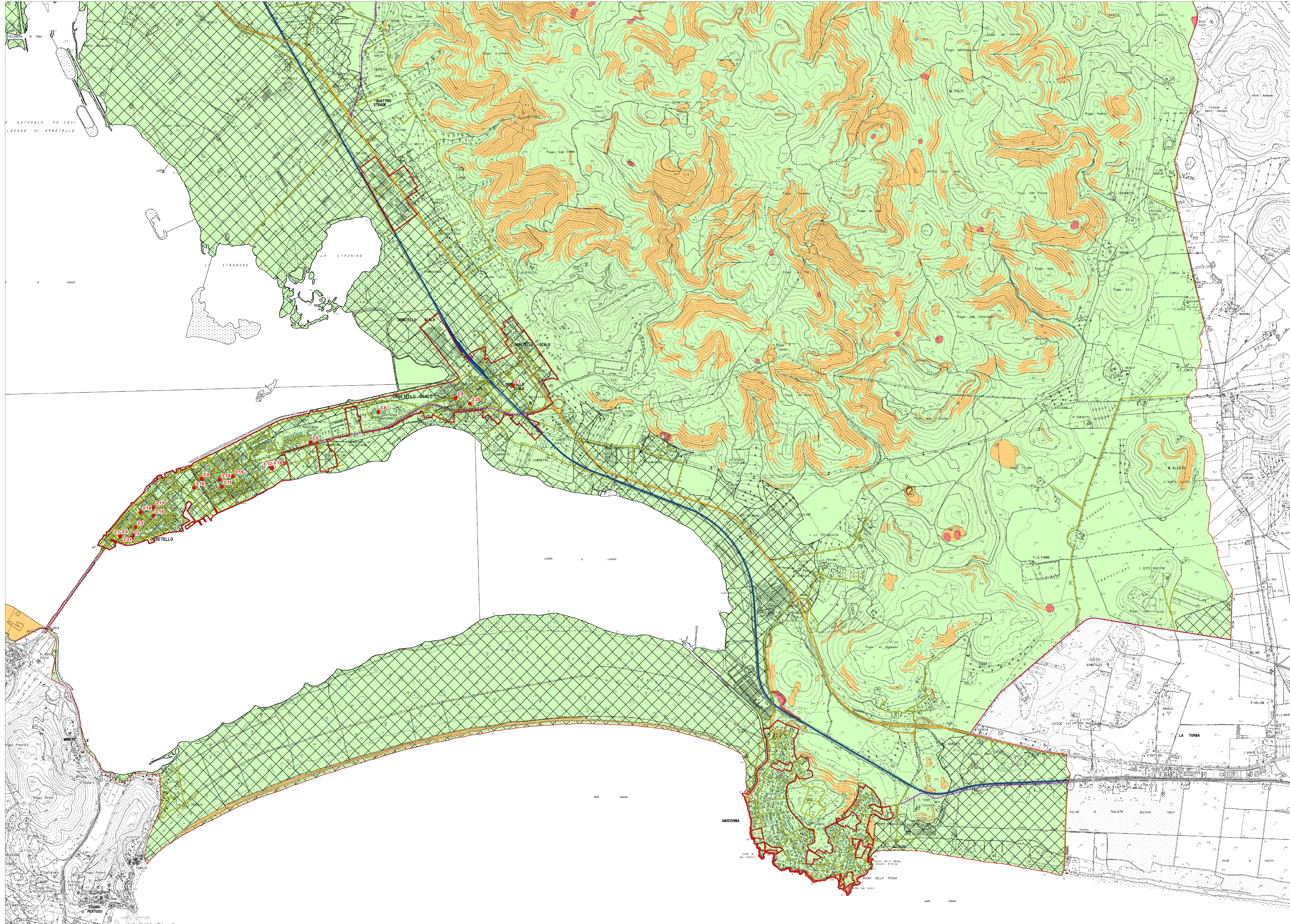
TAVOLA G.01 - Carta delle aree ed elementi esposti a fenomeni geologici
