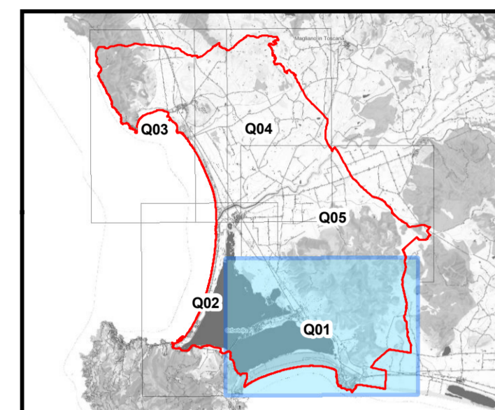
TAVOLA G.01 - Carta delle aree ed elementi esposti a fenomeni geologici
